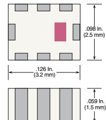
Case 41-2 (EIA 1210 / 3225)
