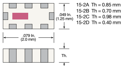
Case 15-2 (EIA 0805 / 2012)
