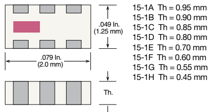
Case 15-1 (EIA 0805 / 2012)
