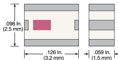
Case 41-1 (EIA 1210 / 3225)
