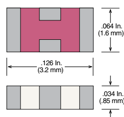
Case 18-2 (EIA 1206 / 3216)
