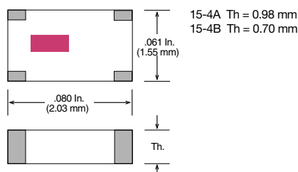
Case 15-4 (EIA 0805 / 2012)
