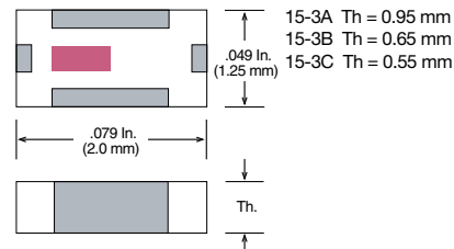
Case 15-3 (EIA 0805 / 2012)
